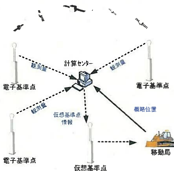
図 2.7 ネットワーク型RTK-GNSS（VRS方式）
